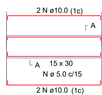
VIGAS (15X30)
