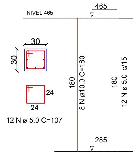
PILARES 30X30
