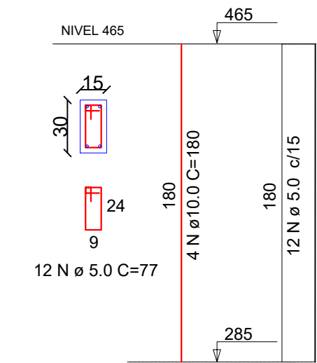
PILARES 15X30
