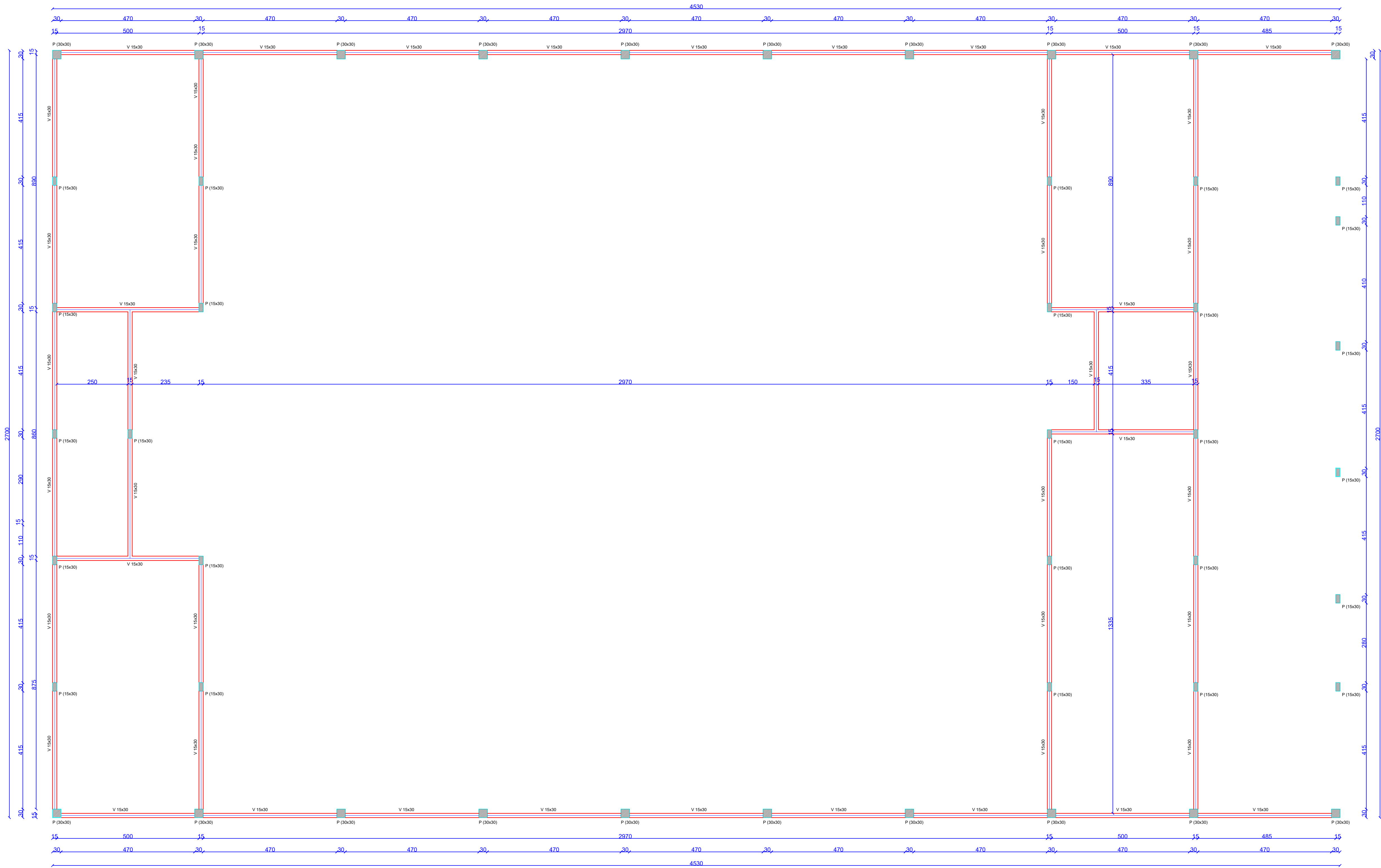
PLANTA DE FORMA DO PAV. COBERTURA (NÍVEL 465)
